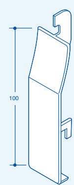
Q117WSB 100mm Shiplap Joint
